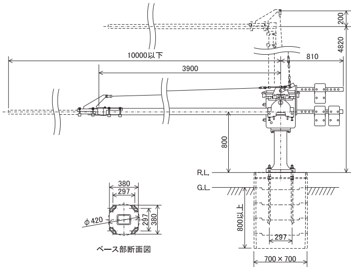
No.18: MCG-ME8F-BDC形外形図 (JR東海事例)
