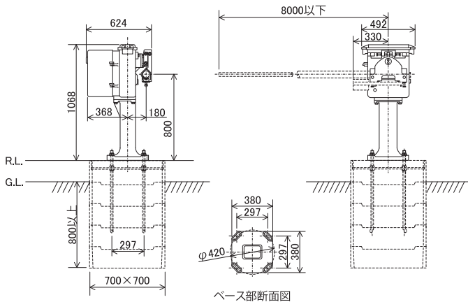
No.15: MCG-ME8F-BC形外形図 (JR東海事例)
